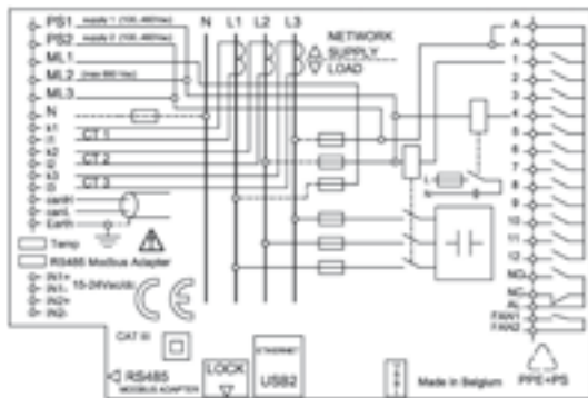
RVT2 3 faz şeması
